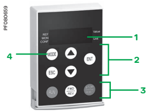
远程显示终端 (盖板打开)
