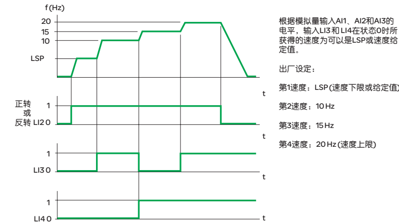
带有4个预置速度和2个逻辑输入的运行示例
