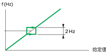
电机速度根据跳频给定值而改变
