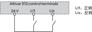
2线控制接线图
