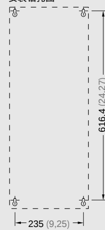
安装钻孔图
