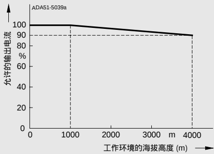
以额定输出电流 % 值表示的 输出电流允许值
