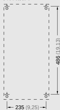
安装钻孔图
