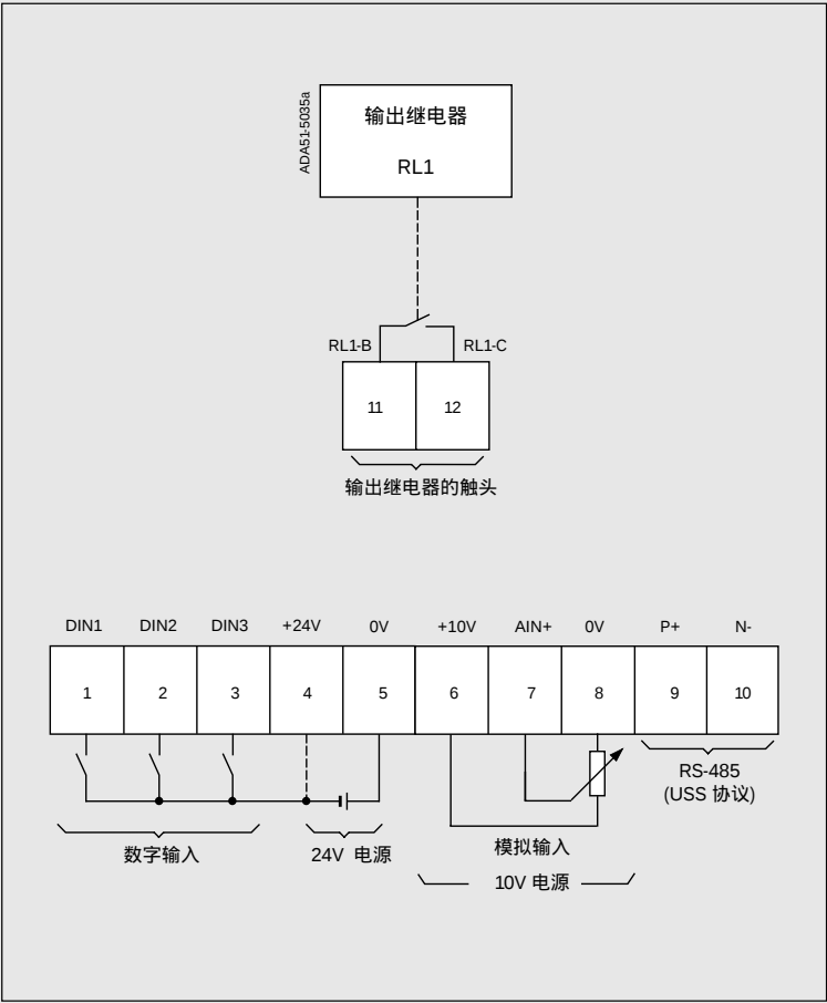
视图 A
