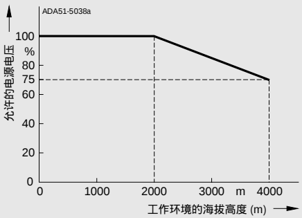
以最大允许电源电压 % 值表示的 电源电压允许值
