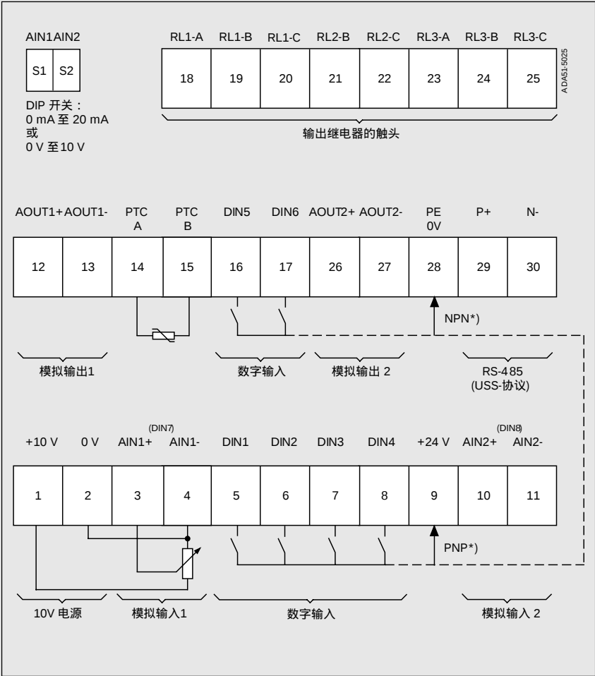
视图 A
