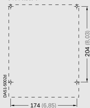
安装钻孔图
