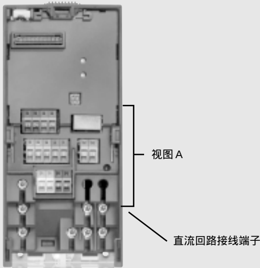
电源接线端子 电动机接线端子
