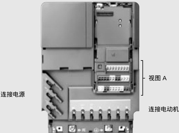
视图 A
