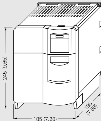
C 型箱体尺寸变频器
