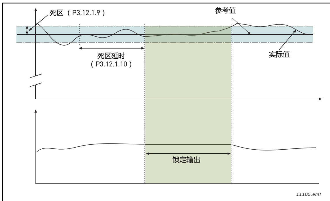
图 33. 死区
