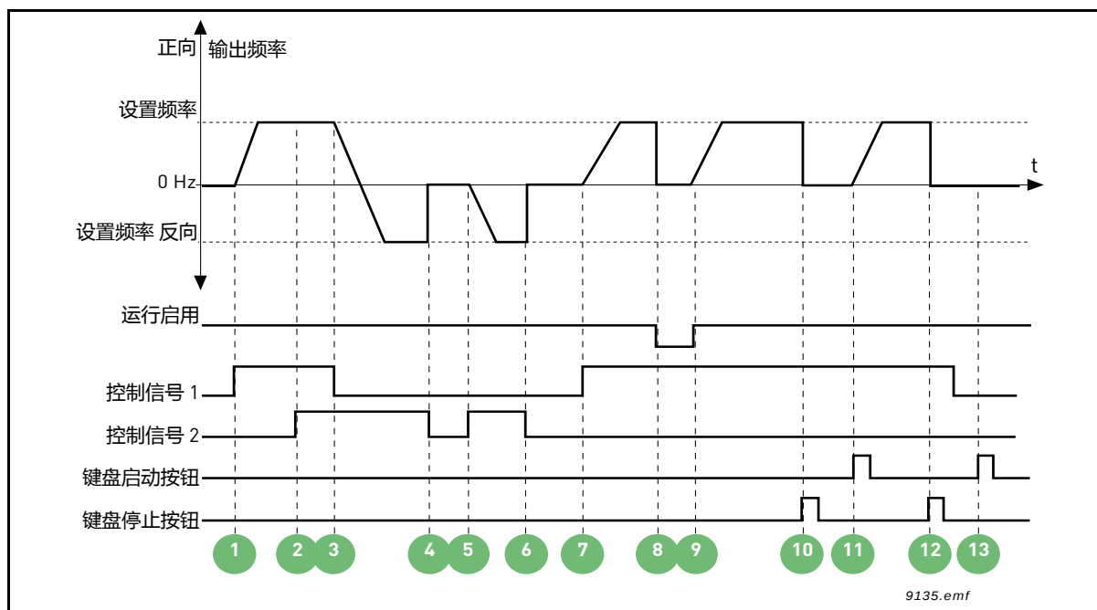
图 19. 正向启动
