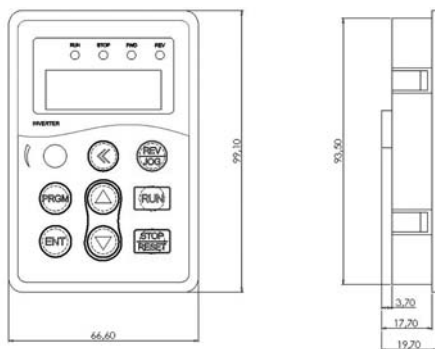
4kW-7.5kW (G) 外引键盘的外形尺寸
