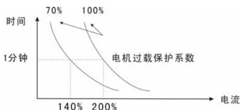
电机过载保护系数设定
