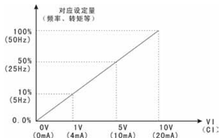
模拟给定与设定量的对应关系
