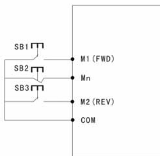
三线式运转模式
