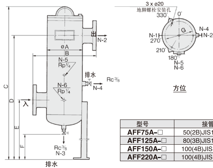
外形尺寸图（毫米）
