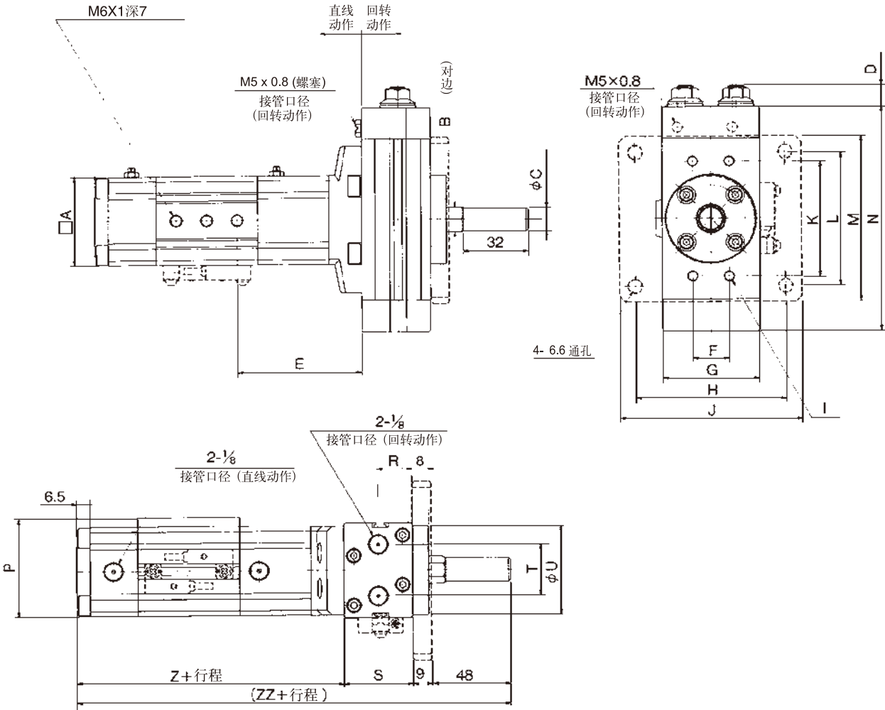
外形尺寸图（毫米）
