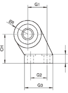
双耳环带耳环座(ES)
