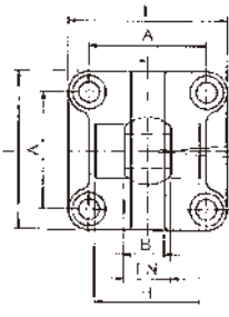
单耳环带耳环座(CS)
