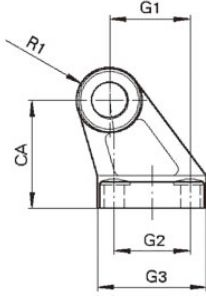
双耳环接座(E)
